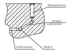
Схема установки дождевателя
